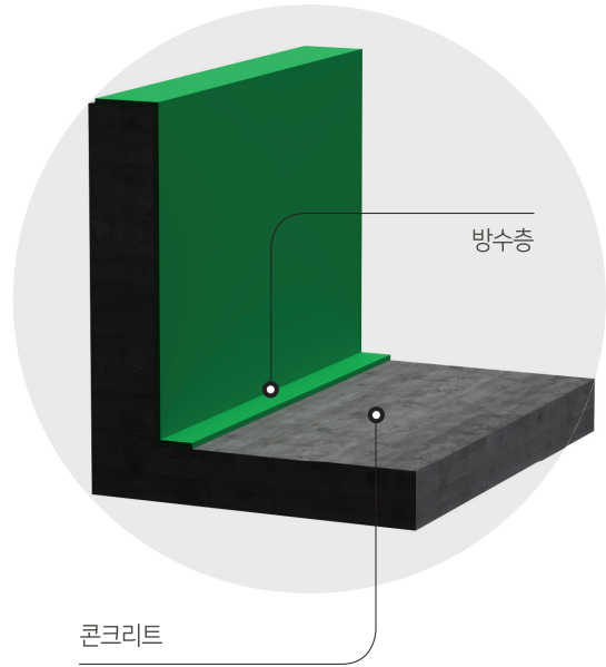
와우플렉스 복합방수공법 수직부 부분
