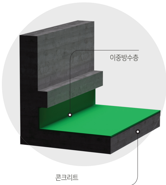
와우플렉스 복합방수공법 모서리 부분
